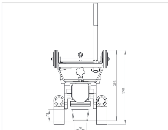
JH 15 G plus | Art.No. 01 150 102-G | Draufsicht | Top view
