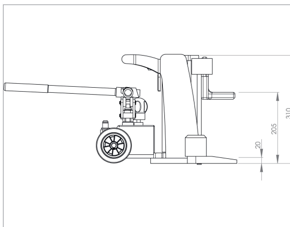
JH 15 G plus | Art.No. 01 150 102-G | Seitenansicht | Side view
